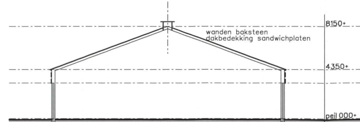
Doorsnede gebouw D
