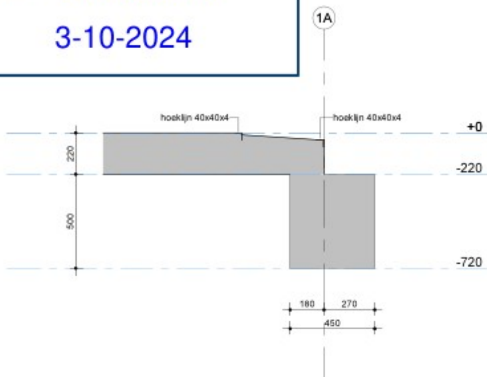
detail A 1 : 20
