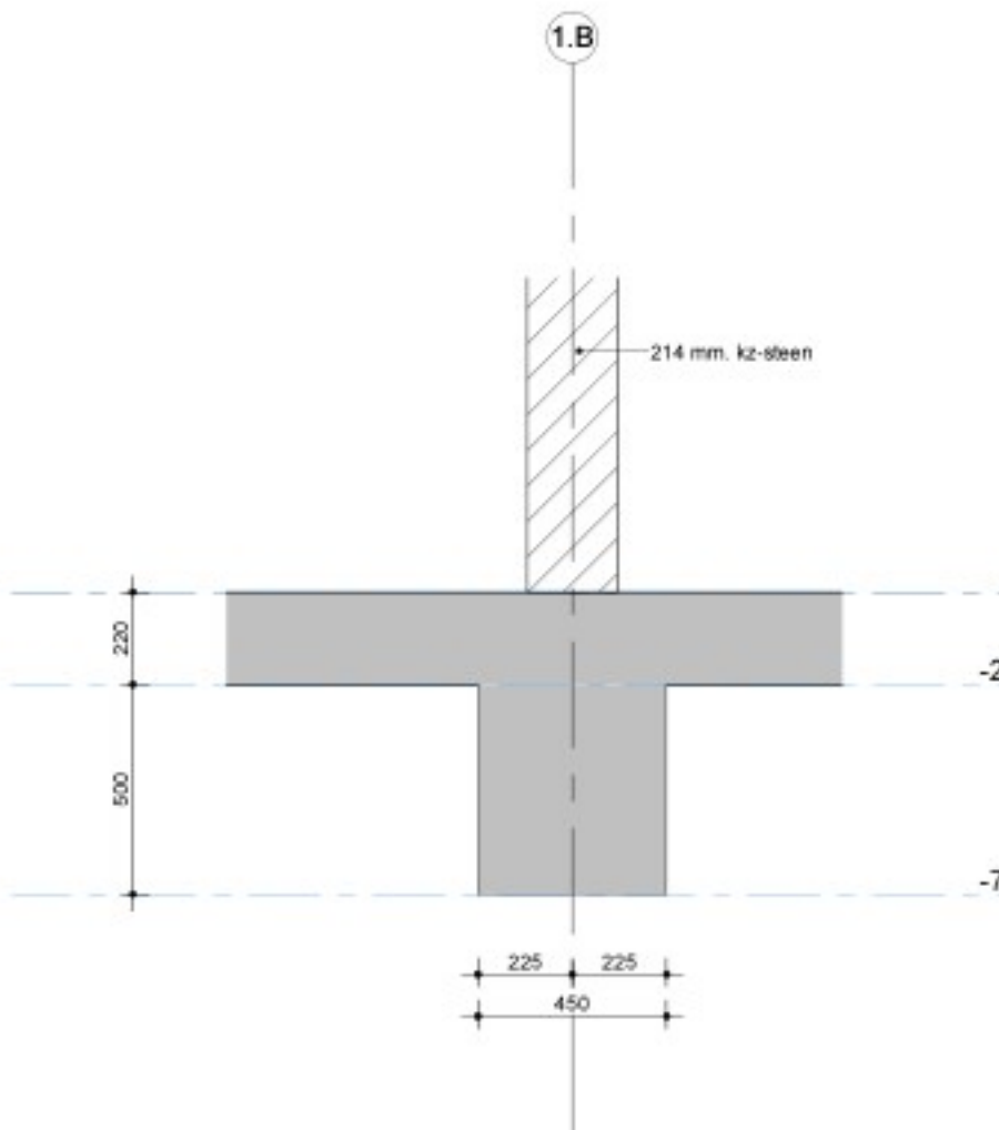
detail B 1 : 20
