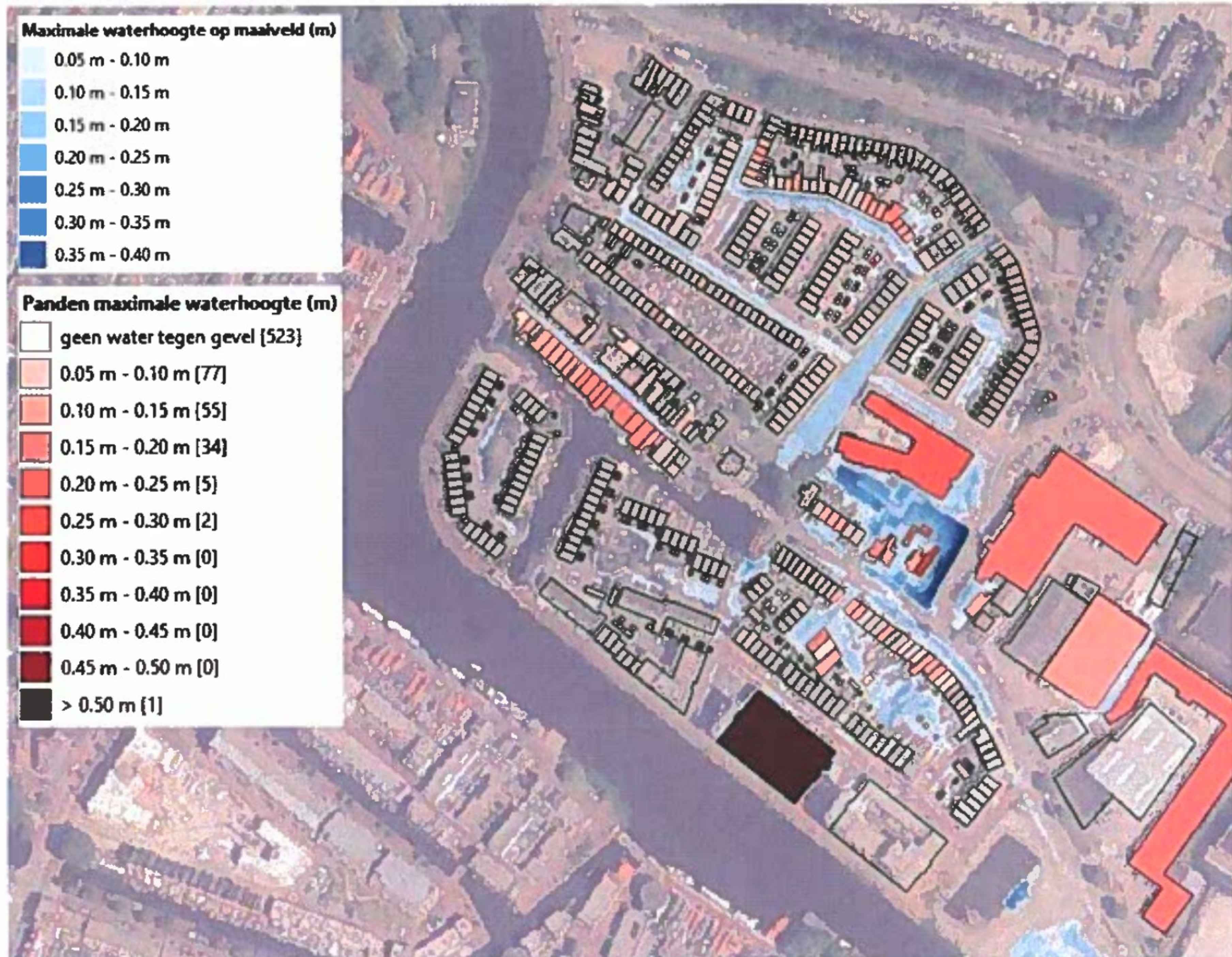
Figuur 24 Overzicht maximale waterhoogte ten opzichte van maaiveld en tegen gevels- toekomstige maaiveldinrichting en huidige rioolstelsels – openbaar gebied – bij 100 mm neerslag in 1 uur
