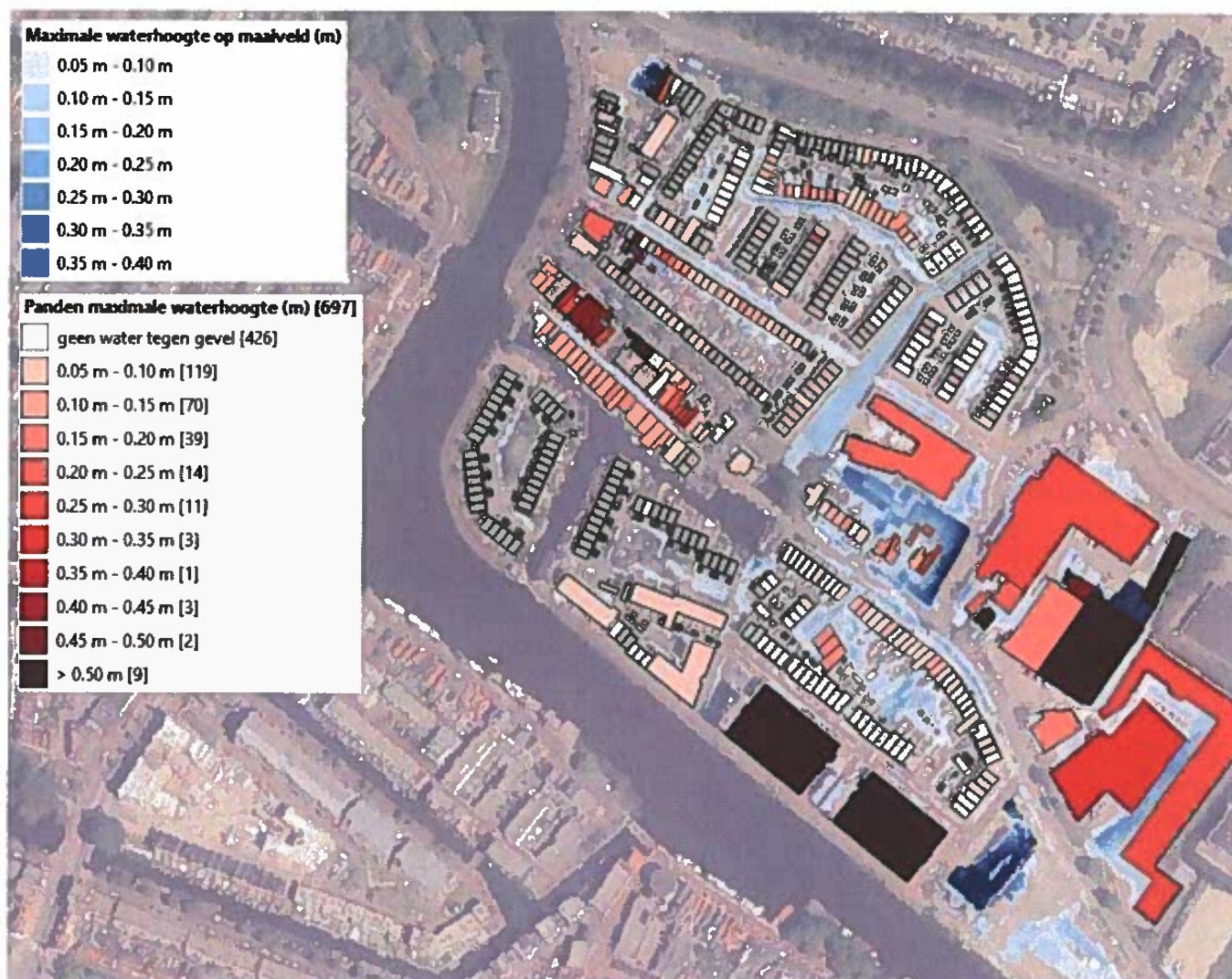
Figuur 23 Overzicht maximale waterhoogte ten opzichte van maaiveld en tegen gevels– toekomstige integrale rioolmodel – openbaar gebied en particulier terrein tezamen – bij 100 mm neerslag in 1 uur
