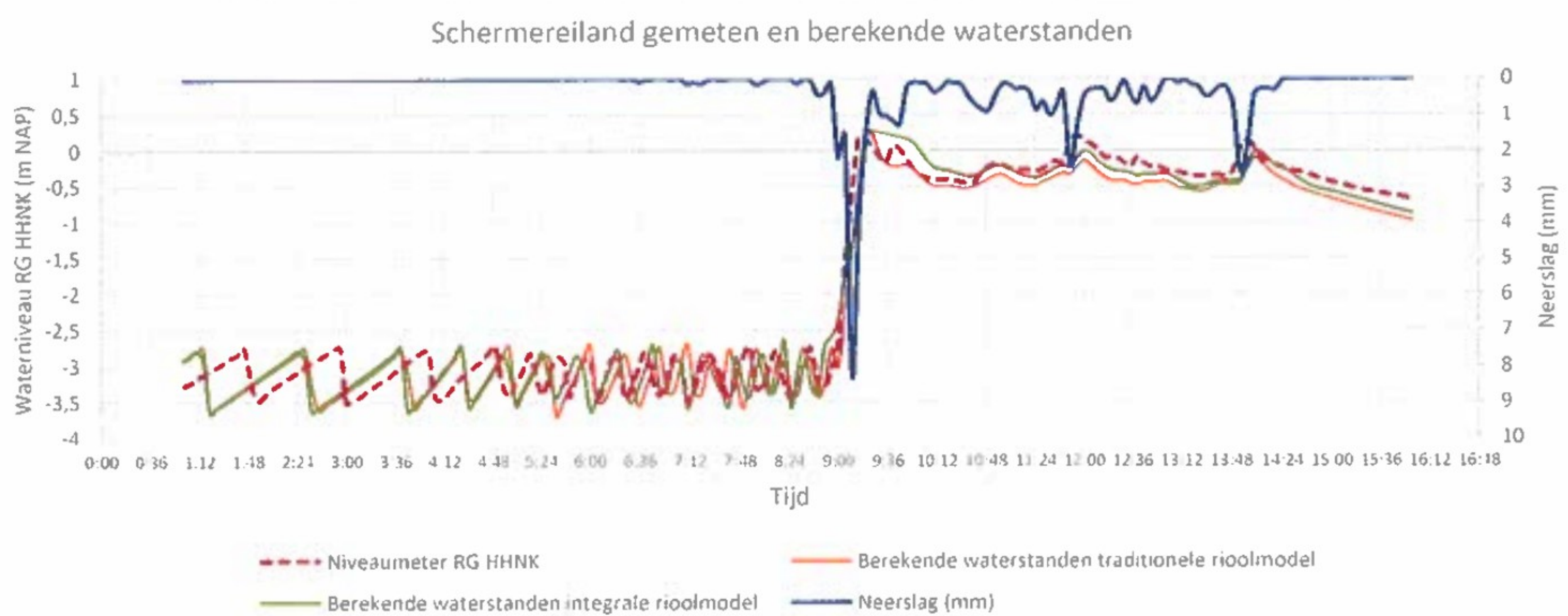
Figuur 13 Schermereiland vergelijking gemeten en berekende waterstanden bij RG HHNK
