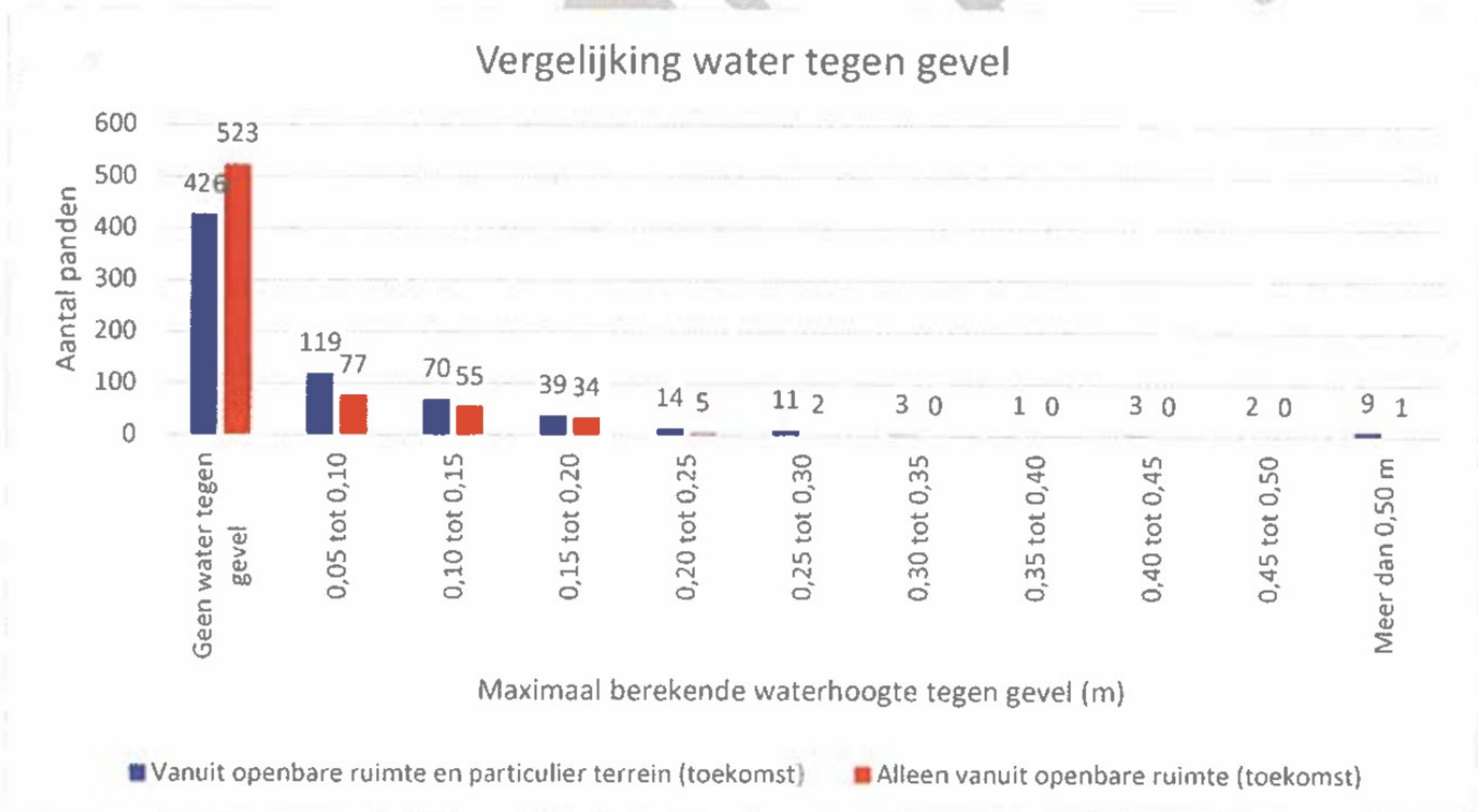
Figuur 25 Toekomstige integrale model: Vergelijking water tegen gevel, openbaar gebied en particulier terrein tezamen versus openbaar gebied
