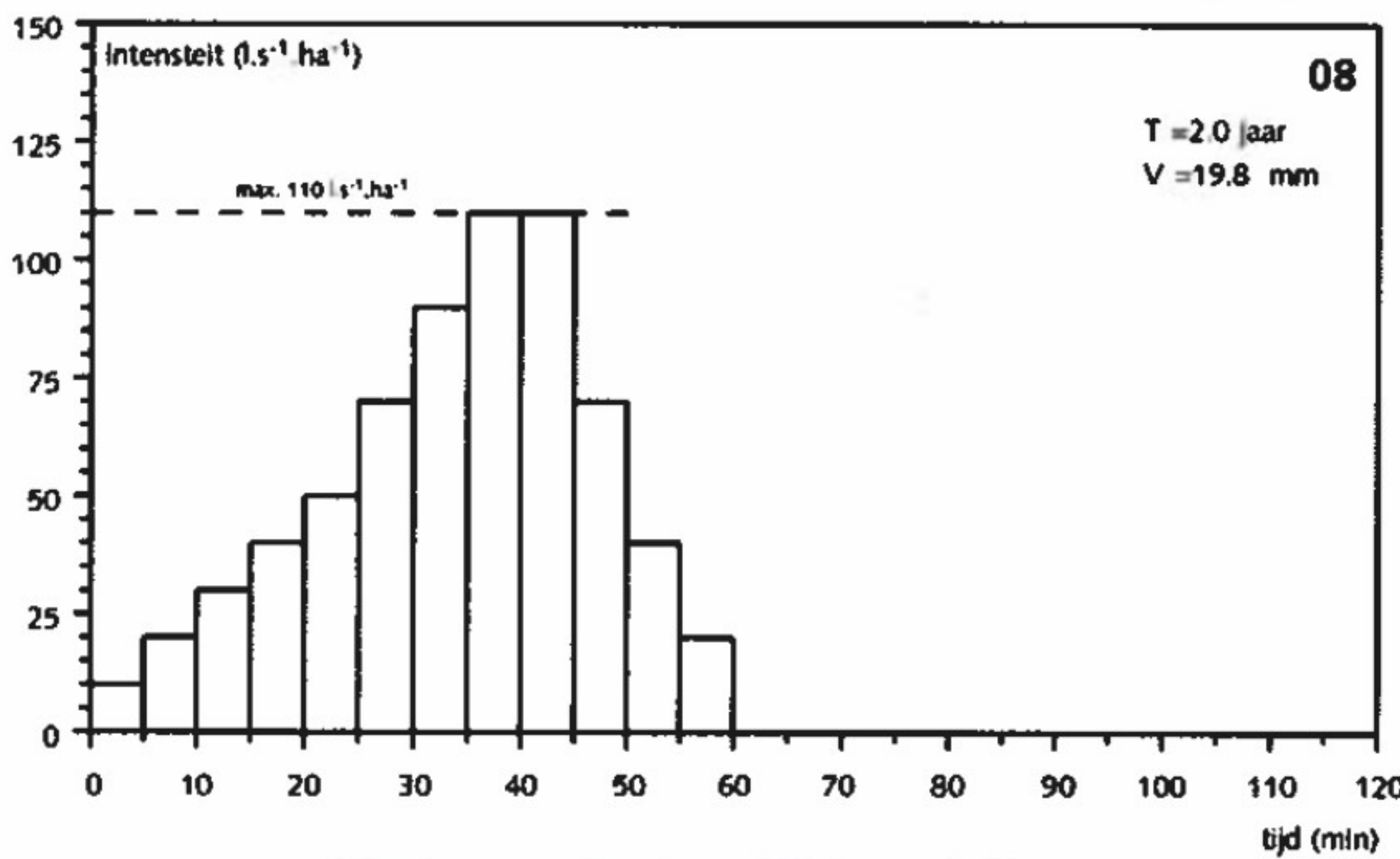
Figuur 3 Neerslaggebeurtenis BUI8, grafische weergave verloop neerslaggebeurtenis
