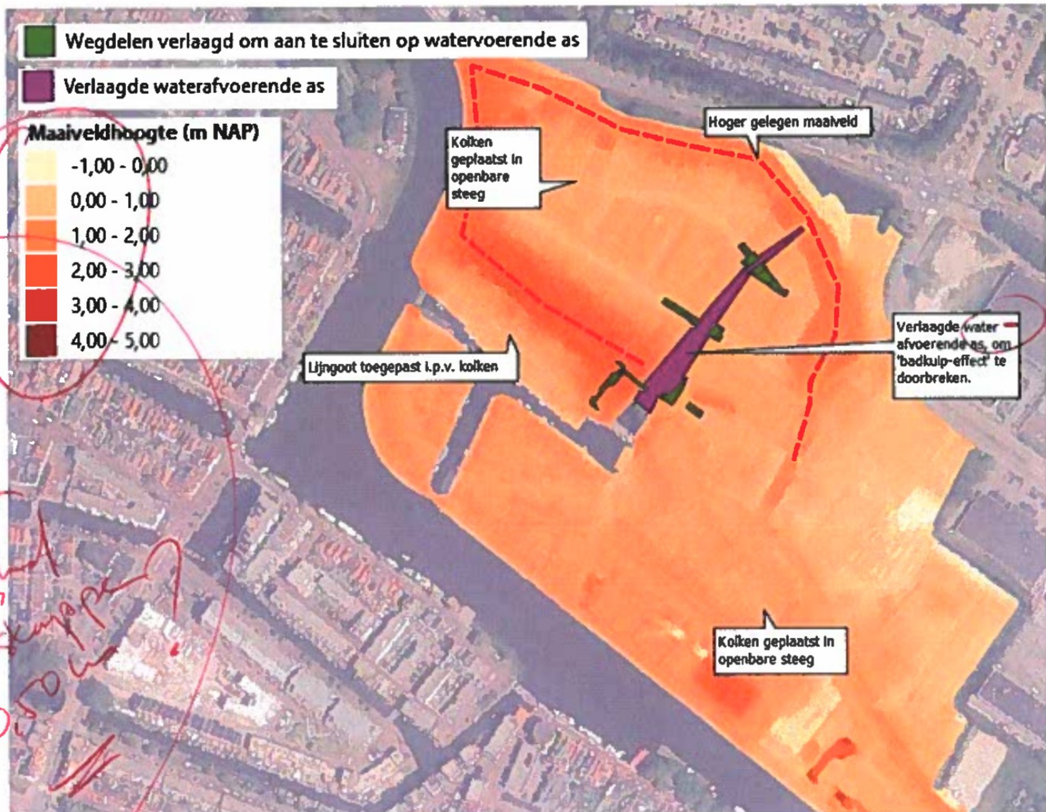
Figuur 22 Maaiveldmodel, overzicht doorgevoerde aanpassingen
