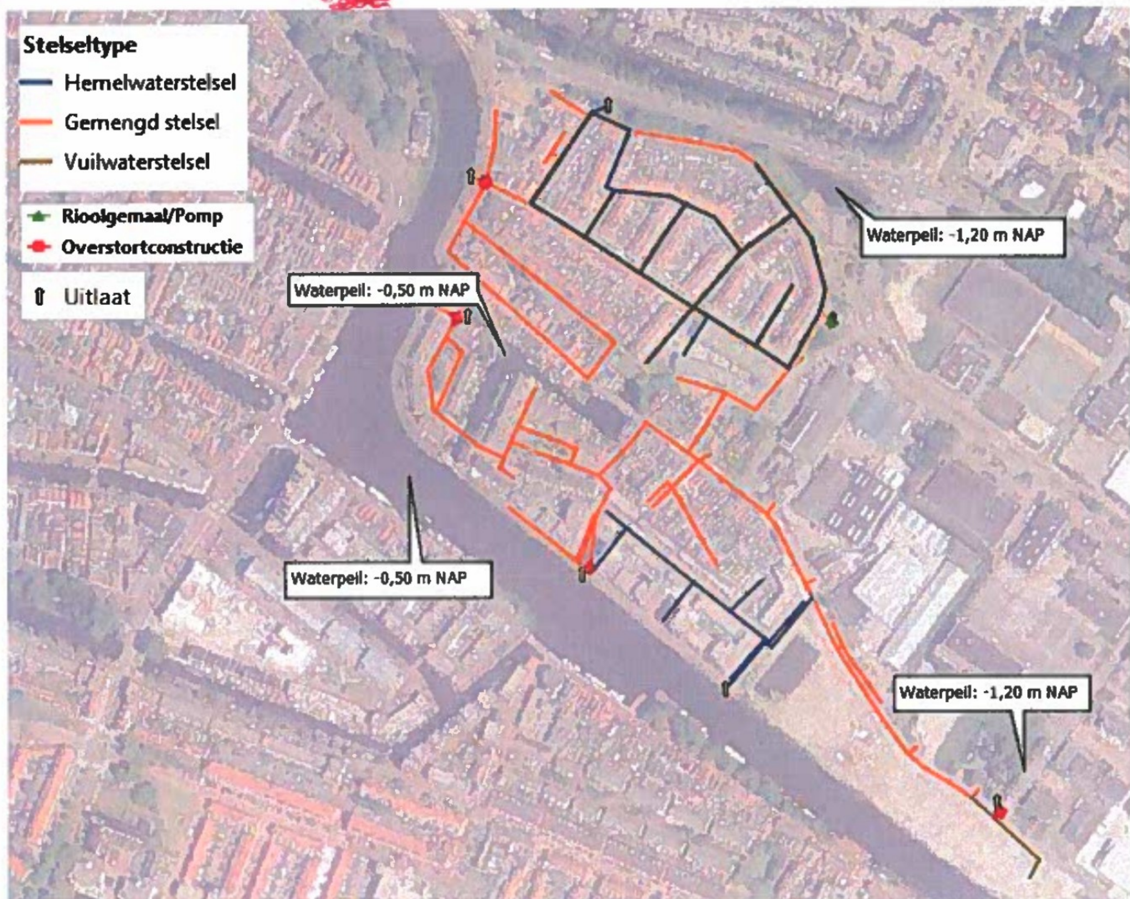
Figuur 2 Leidingtypen en oppervlaktewaterpeilen binnen projectgebied
