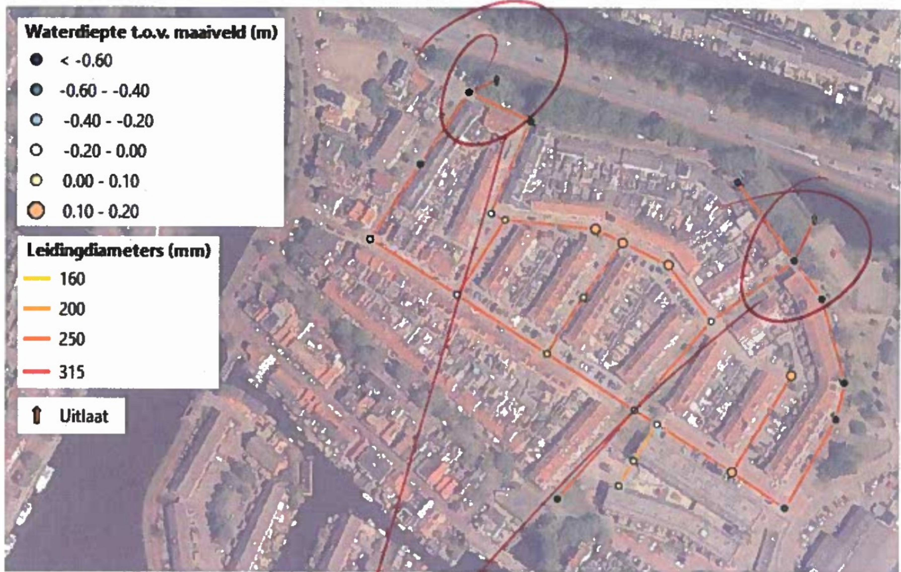
Figuur 21 Mogelijke toekomstige hemelwaterstelsel functioneren bij neerslag 9 oktober 2019
