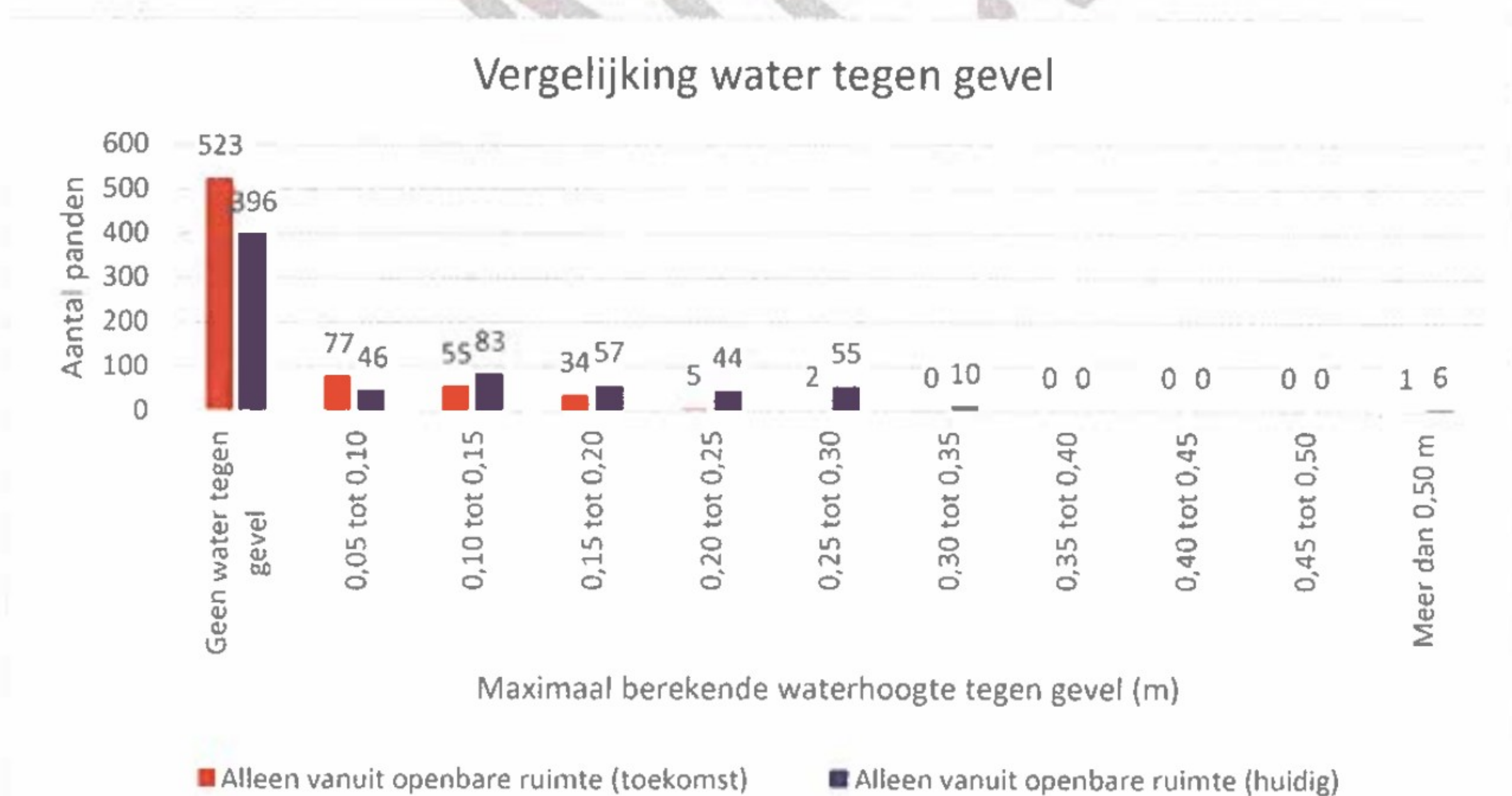
Figuur 28 Vergelijking maximale waterhoogte tegen gevels van uit openbaar gebied – heden versus toekomstige integrale rioolmodel
