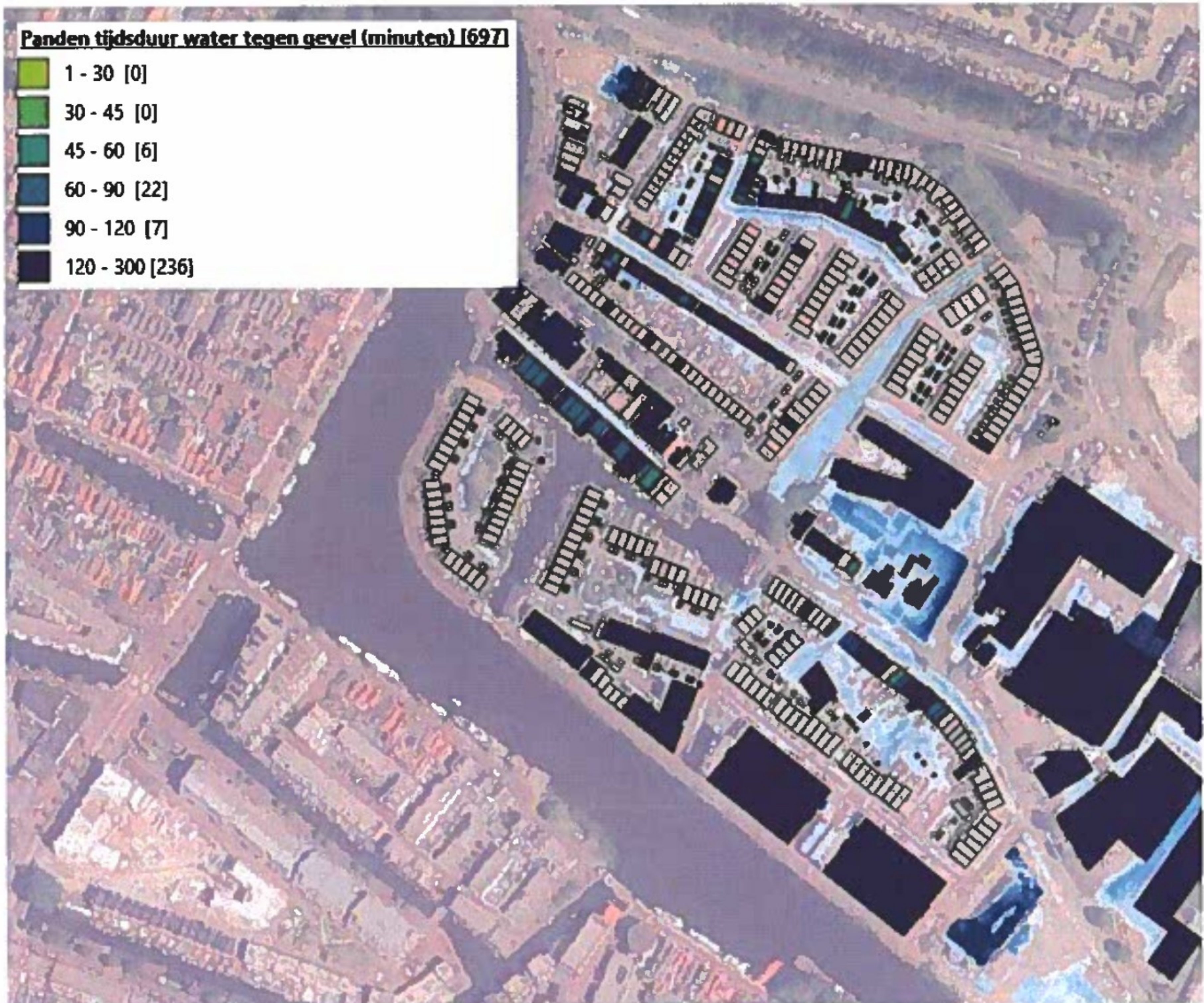
Figuur 26 Overzicht tijdsduur water tegen gevels – toekomstige integrale model – openbaar gebied en particulier terrein tezamen – bij 100 mm neerslag in 1 uur
