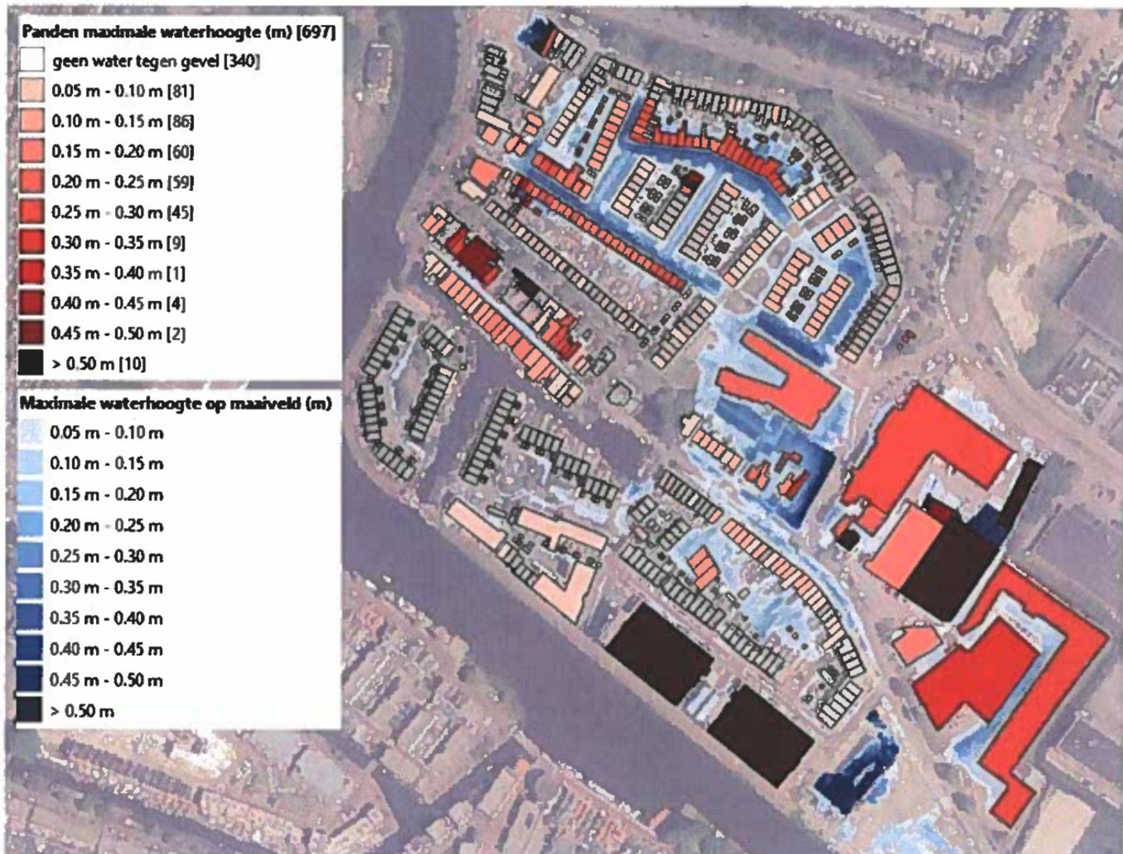
Figuur 16 Overzicht maximale waterhoogte ten opzichte van maaiveld en tegen gevels – huidige maaiveldinrichting en huidige rioolstelsels – openbaar gebied en particulier terrein tezamen – bij 100 mm neerslag in 1 uur
