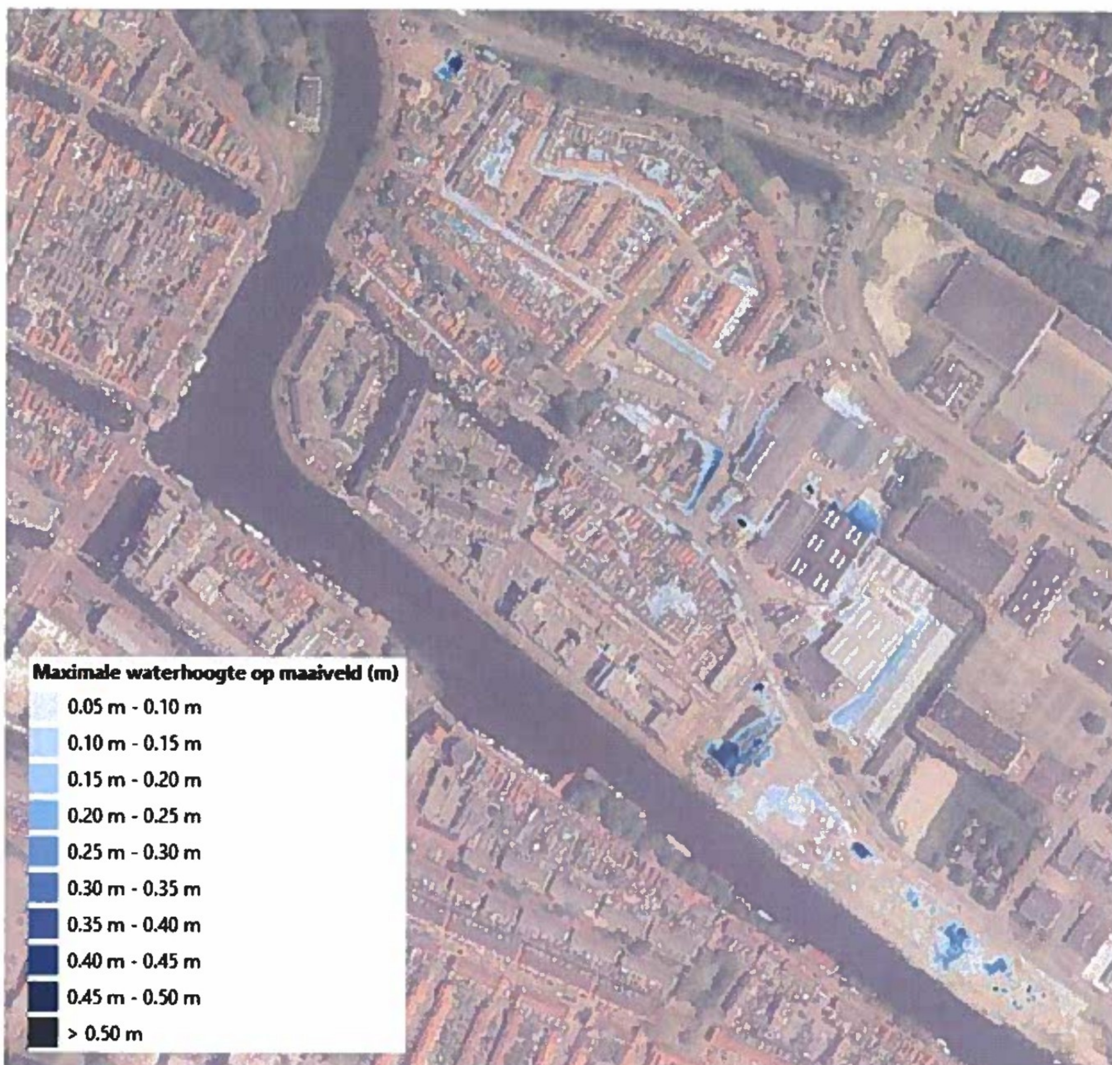
Figuur 12 Huidige rioolstelsels in combinatie met maaiveldmodel, maximaal berekende omvang en waterhoogte van water op maaiveld
