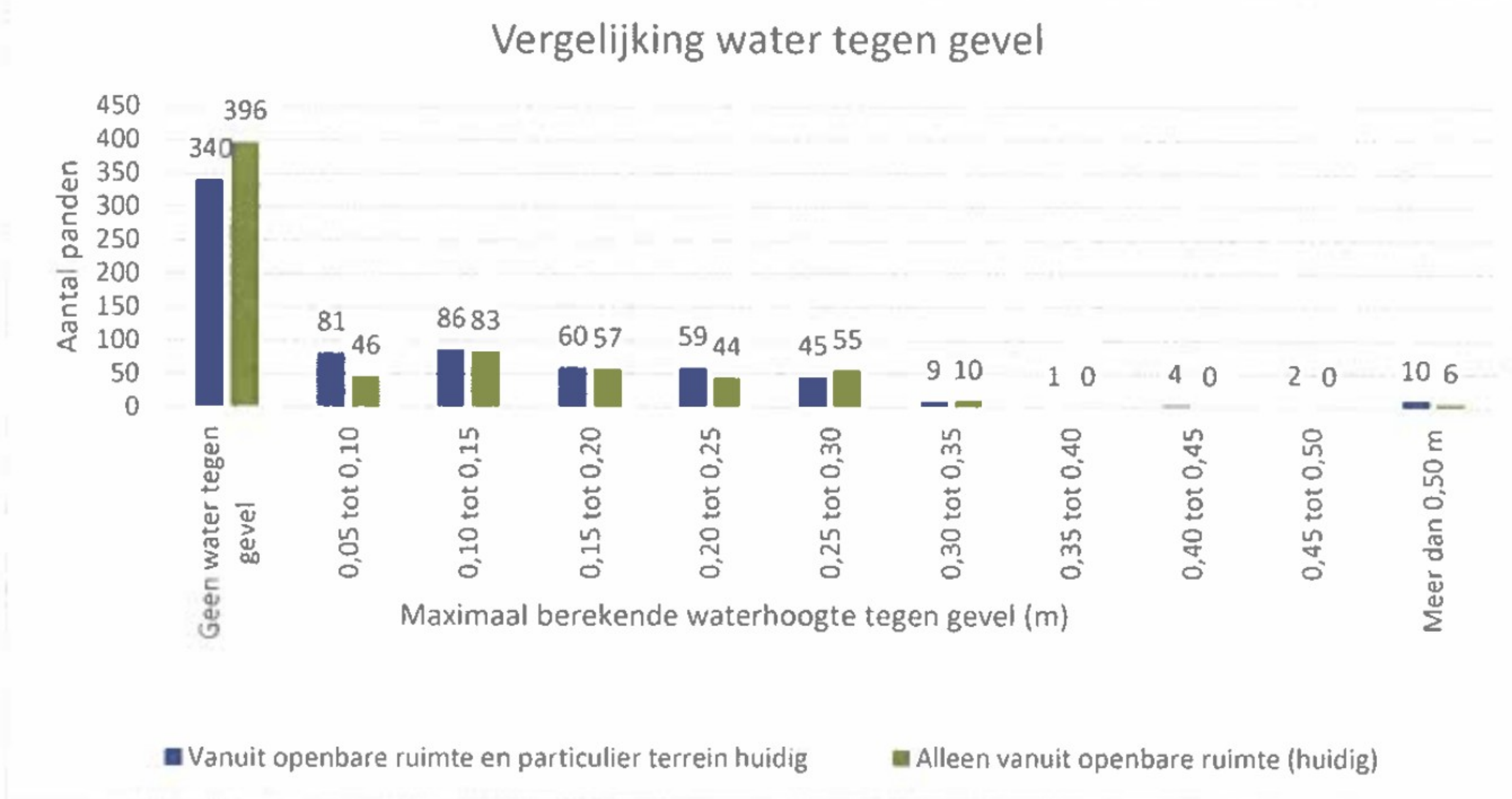
Figuur 18 Vergelijking water tegen gevel openbaar gebied en particulier terrein tezamen versus openbaar gebied 5
