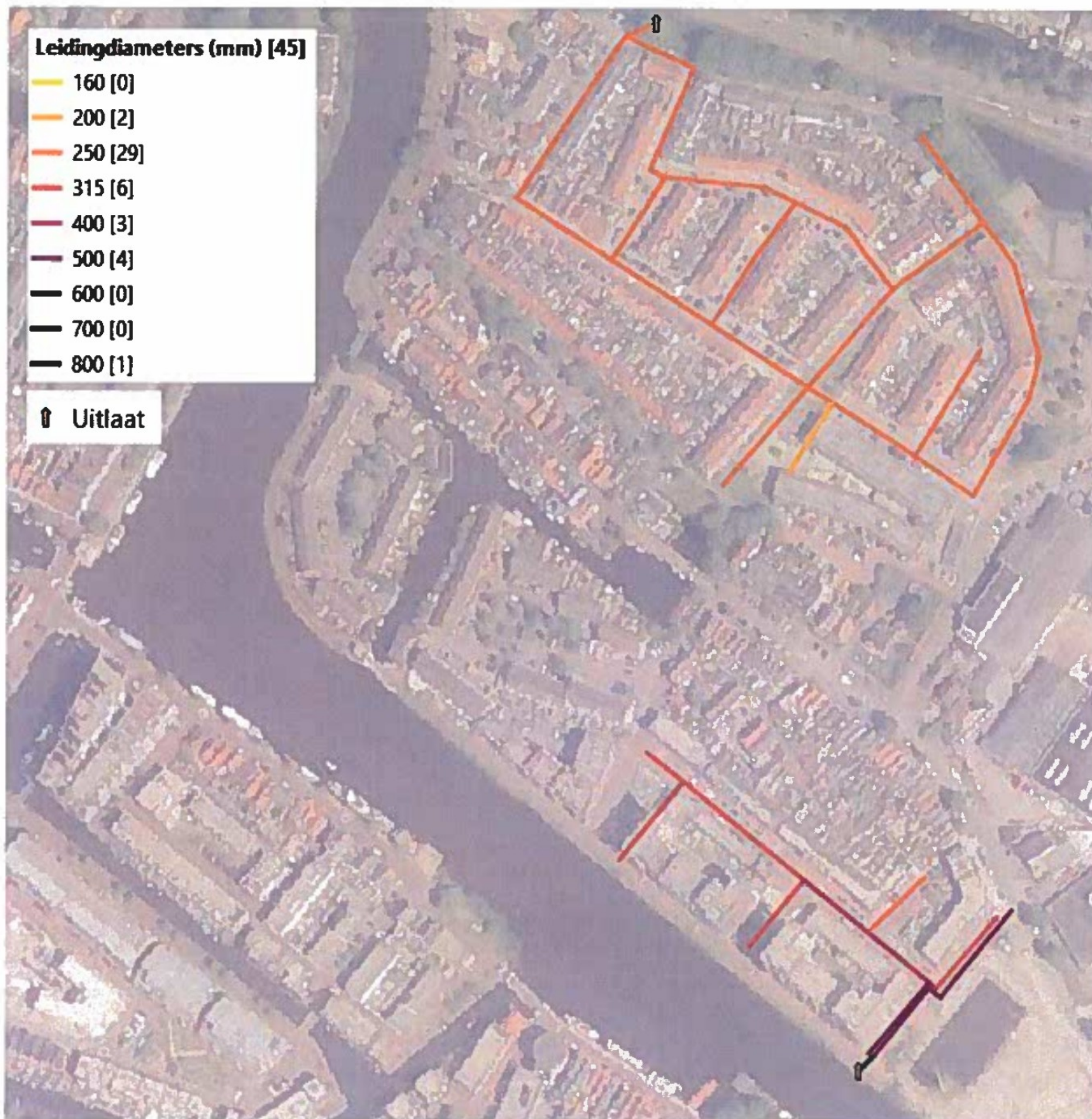
Figuur 9 Overzicht hemelwaterstelsels, binnen projectgebied
